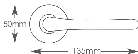
Satin Nickel IH-ATL.09.SNP
